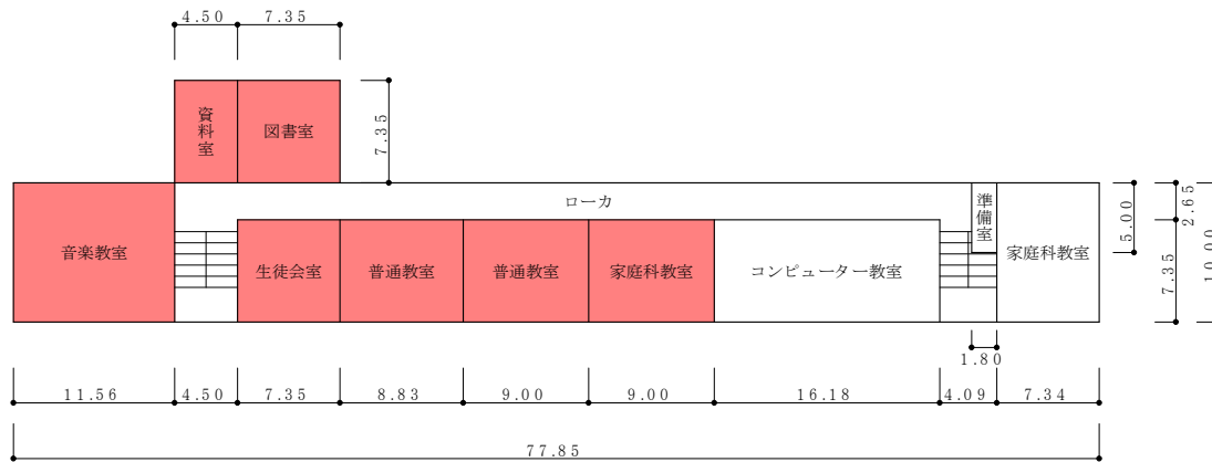
2階平面図
